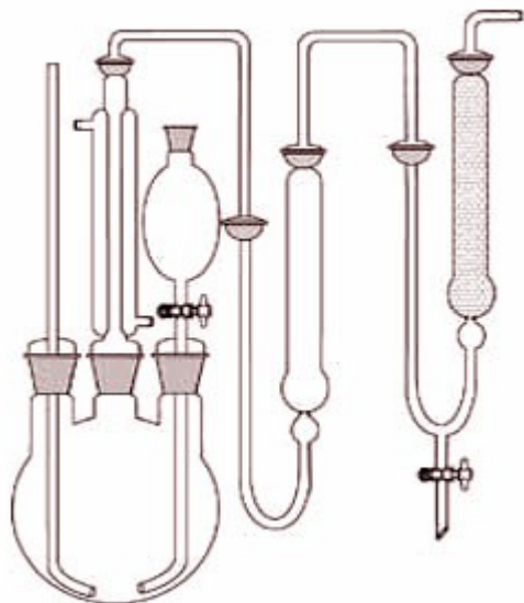
APPARECCHIO X LA DETERMINAZIONE DITIOCARBAMMATI
