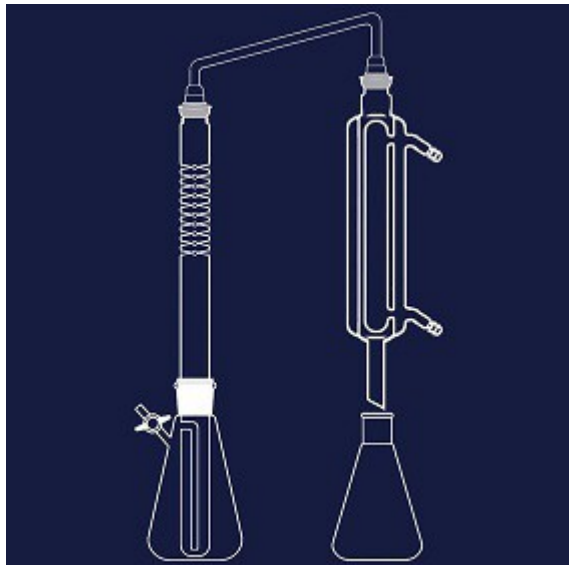
ACIDIMETRO CAZENAVE-MICONI SOLO VETRO
